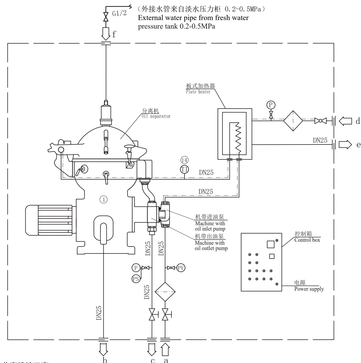
> 分离机接口表 Separator Interface Table
