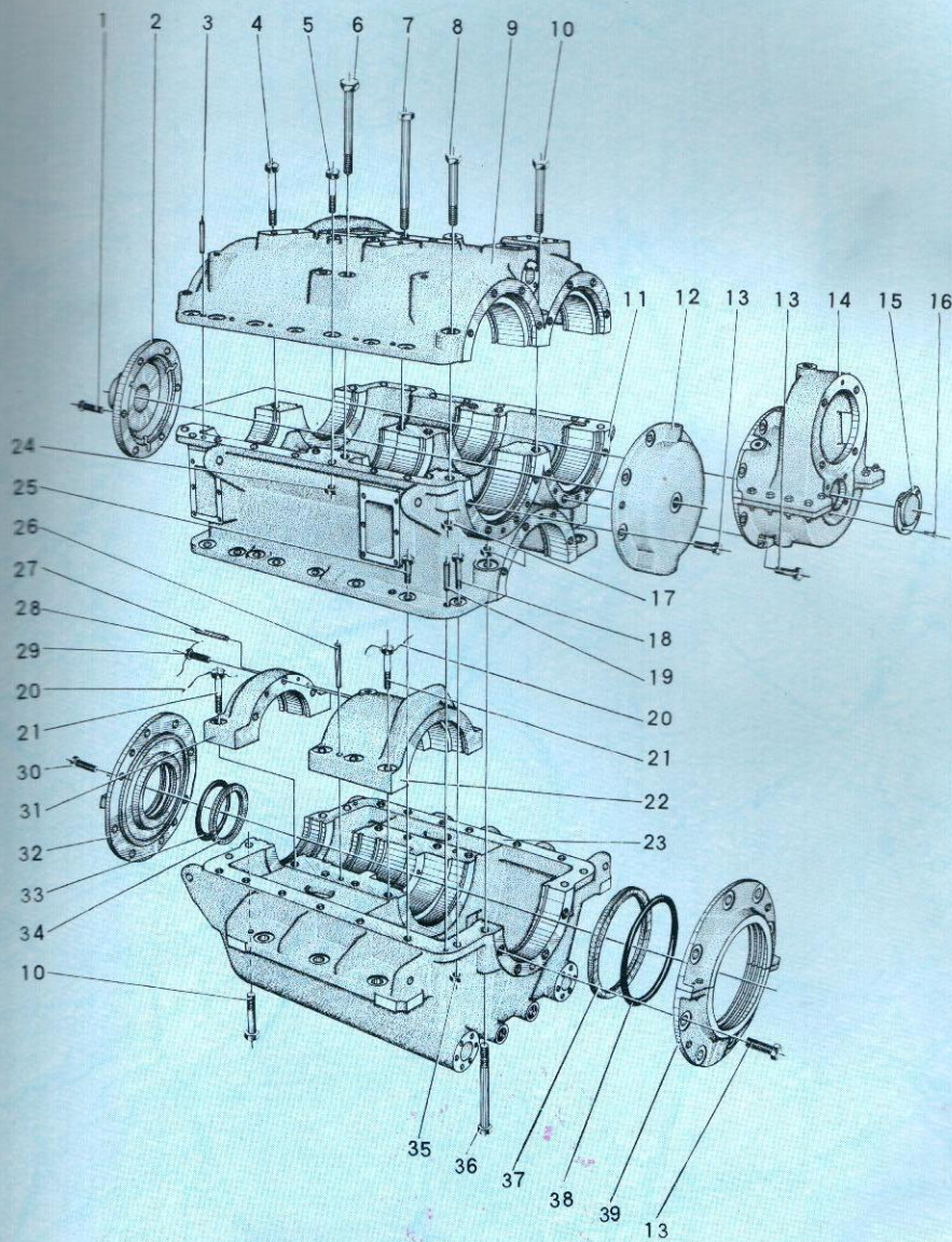
4. 箱 体 Gear casing
